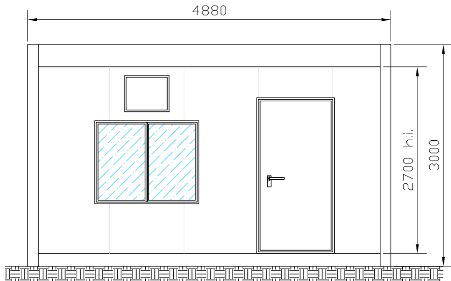
PROSPETTO LATO A
