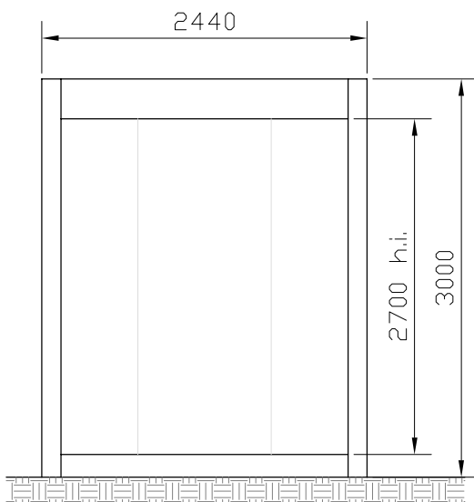
PROSPETTO LATO C
